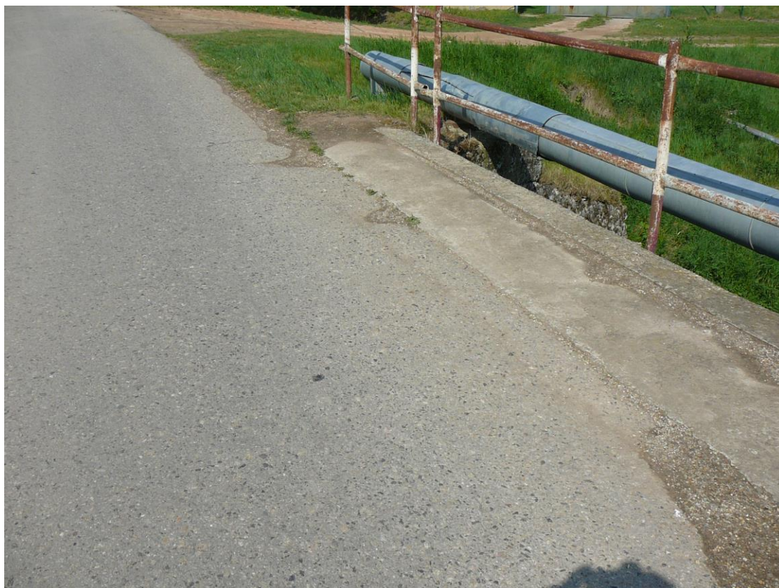
13. Pohľad na rímsu a vozovku – vtoková strana
